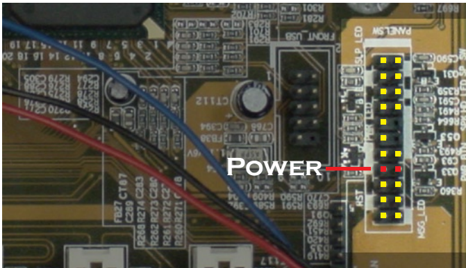
PWR_BTN
